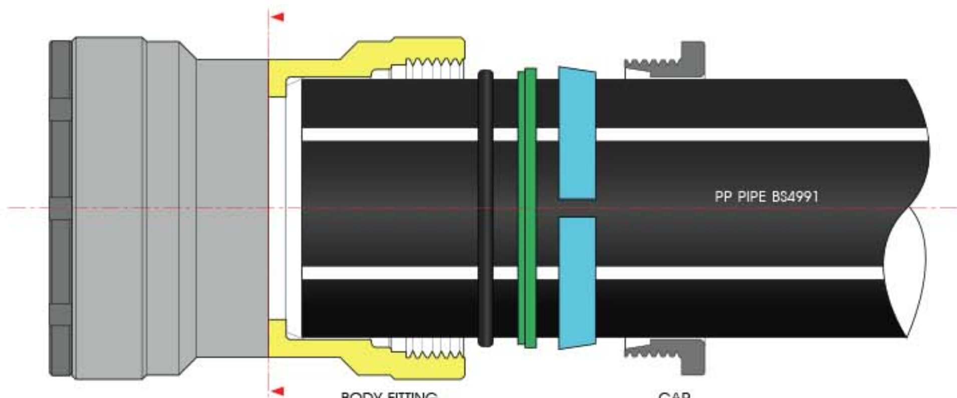
การจัดเรียงชิ้นส่วน ติดตั้งท่อพีพี 150 - 250 มม.
